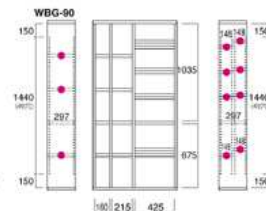
書棚(限定) WBG-90 本体価格 ¥36,300 ホワイト・グレー W900 D300 H1800mm プリント化粧板 ●棚板:大3枚、小3枚、右部前後棚8枚 ●固定金具 4528793007335
