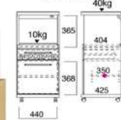
レンジ台 ARA-48
