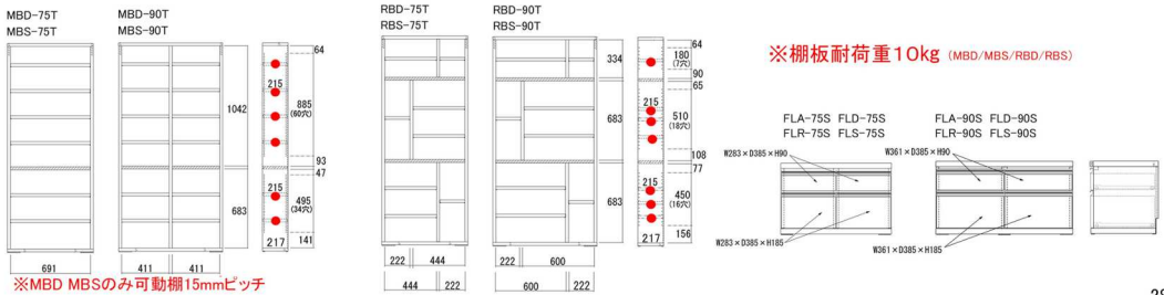
ランダムシェルフ RBS-75T ¥42,020 (税抜価格) ¥38,200 ホワイトウッド W743 D221 H1800mm プリント化粧板 ●棚板大5枚 小3枚 ●固定金具 4528793008790
